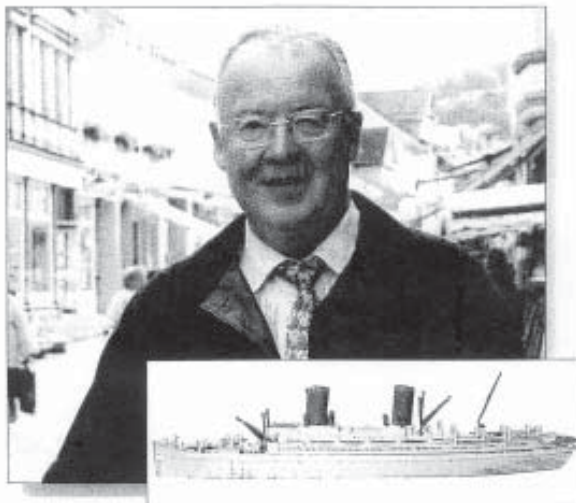
001-1230 Der Allenburger Frank-Rainer Köpke mit dem Modell der „Steuben“.
